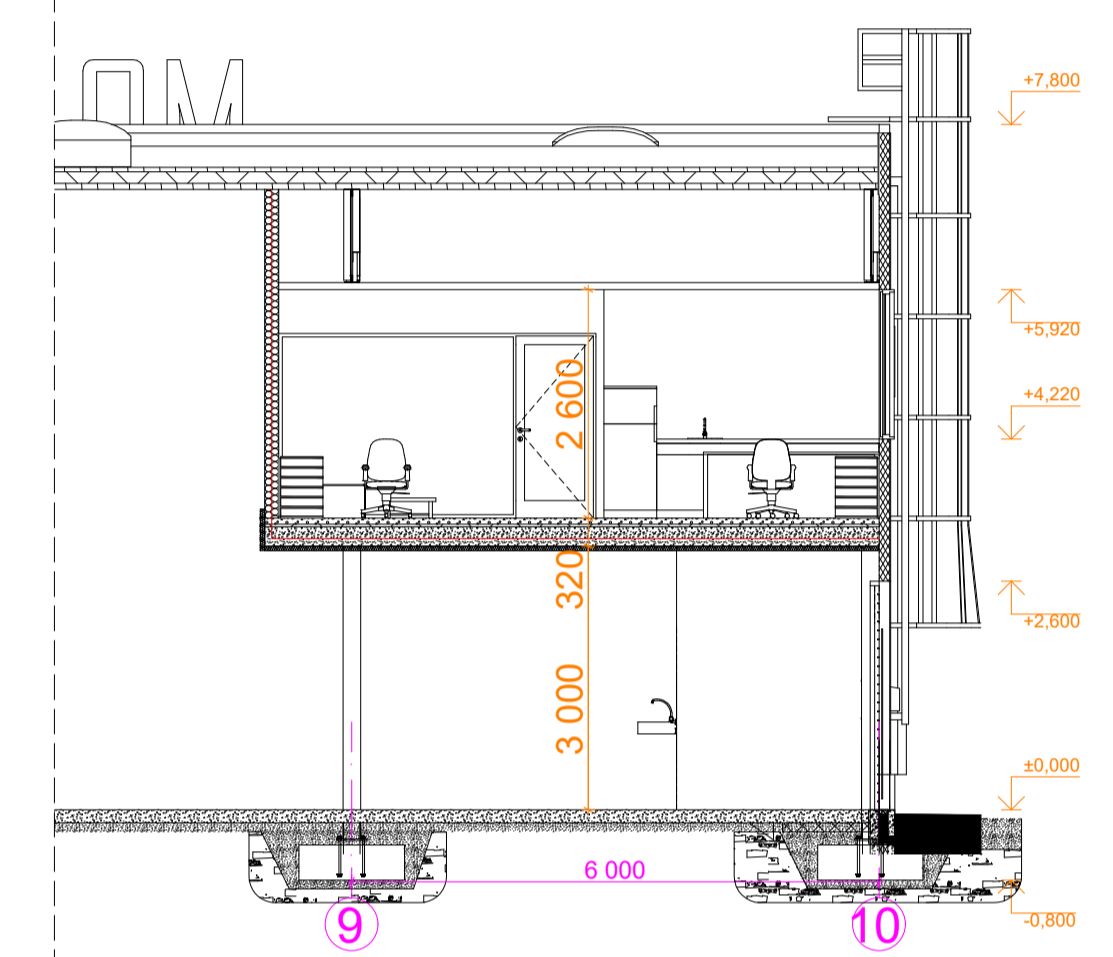
MÄEKÜLA TN 9 | LÕIGE L-3
