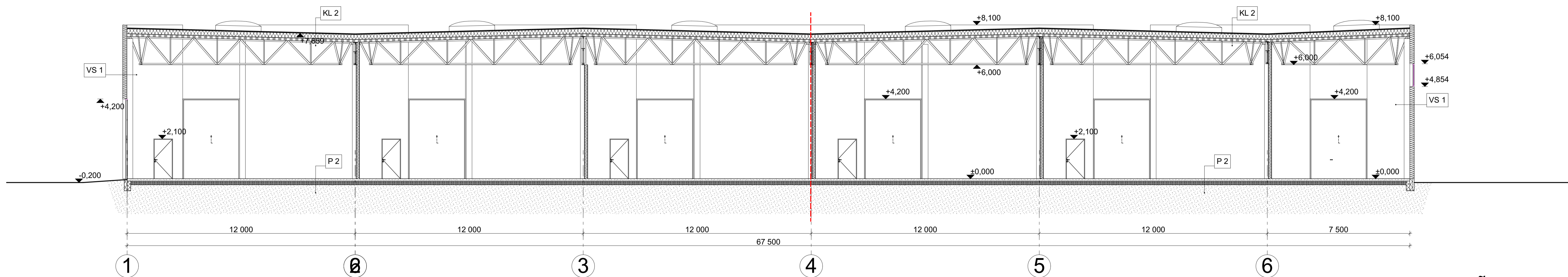
LÕIGE 2-2
